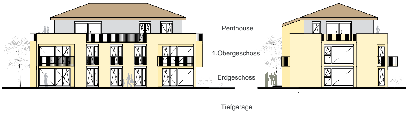
Ansicht Südost - Gartenseite
